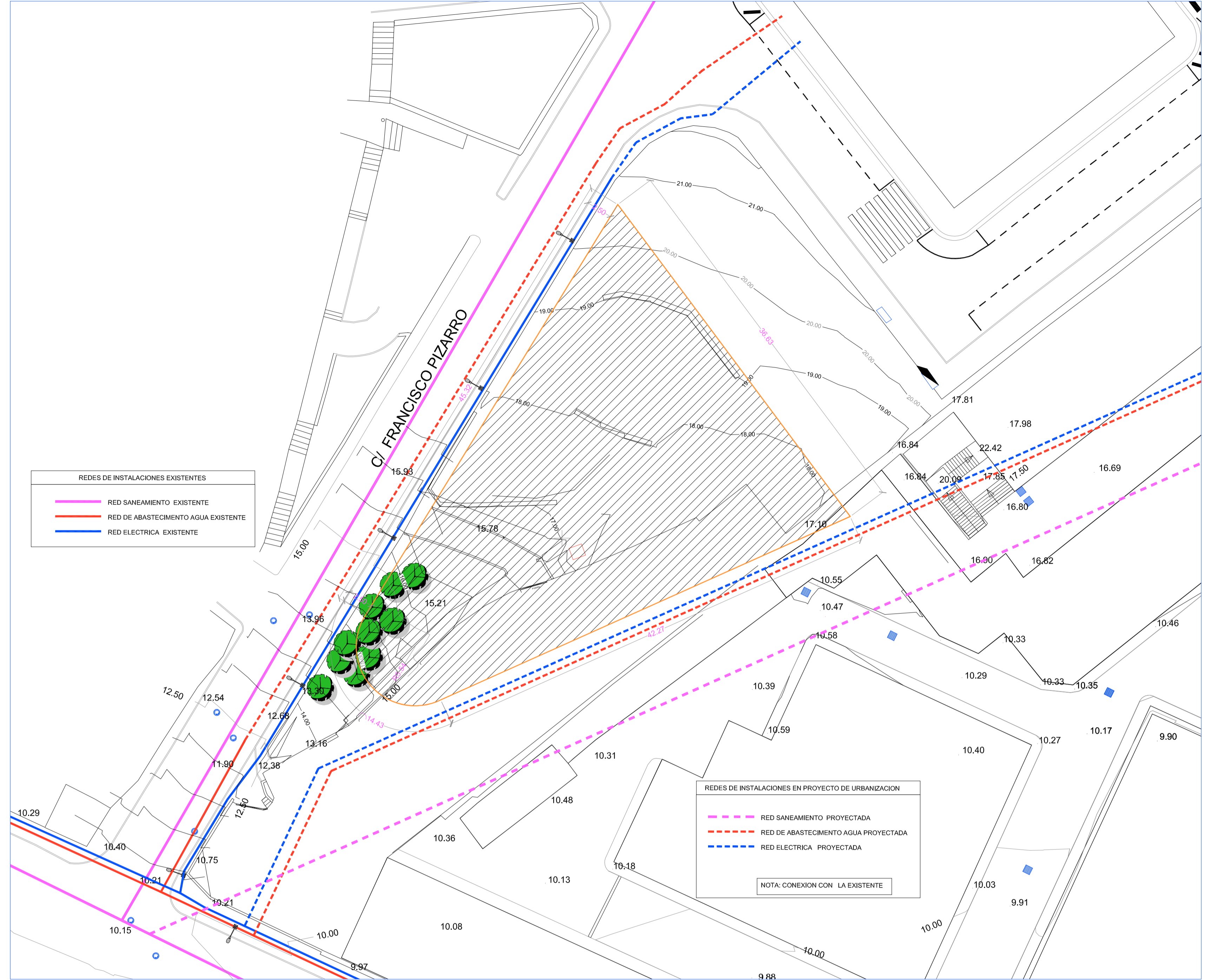
ESTADO ACTUAL Y REDES DE INSTALACIONES URBANAS Escala 1/250
