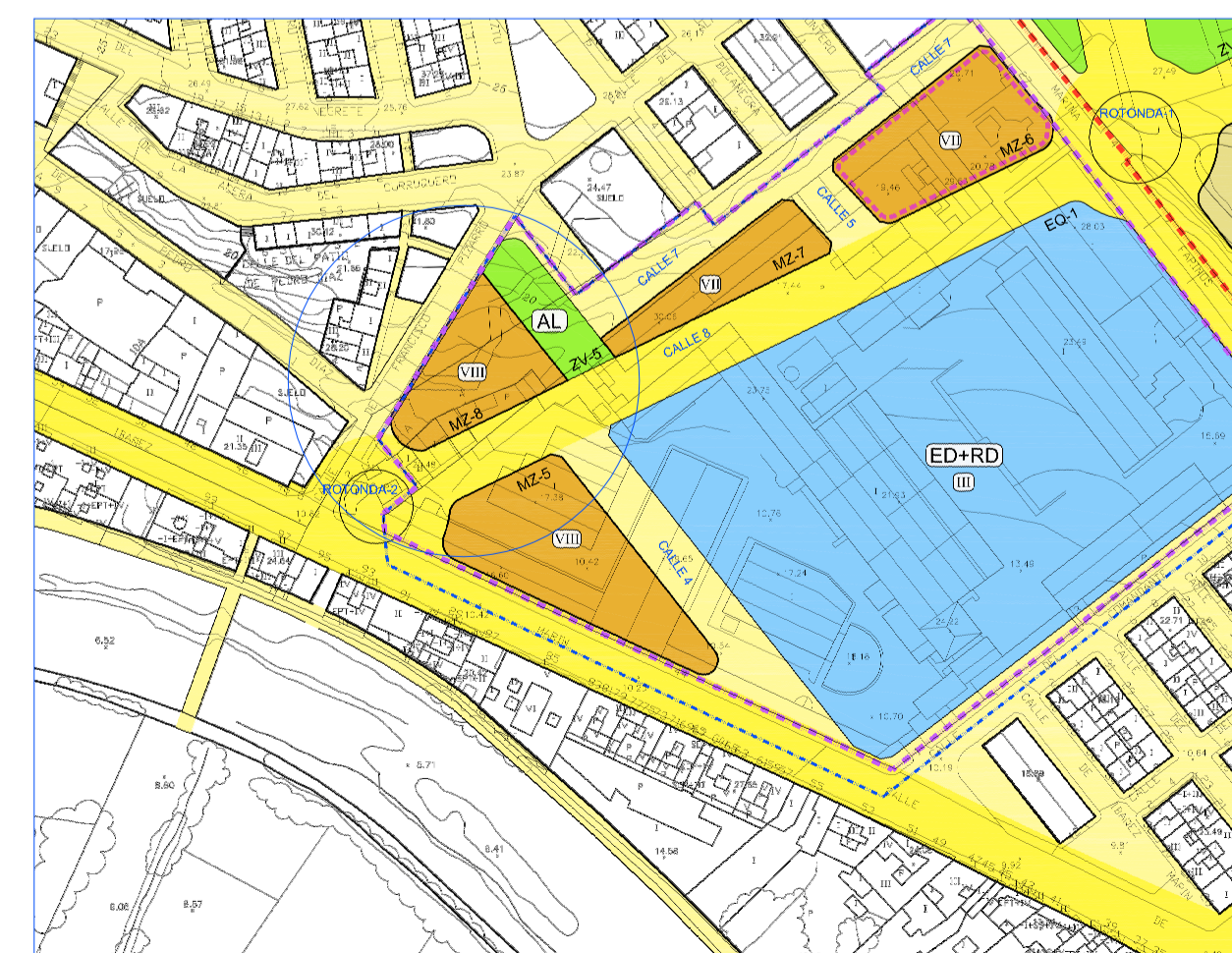
SITUACION EN EL PGOU Escala 1/2000
