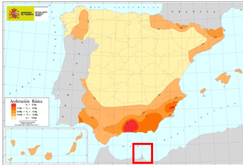
Figura nº 13: Aceleración sísmica básica en España (IGN).
