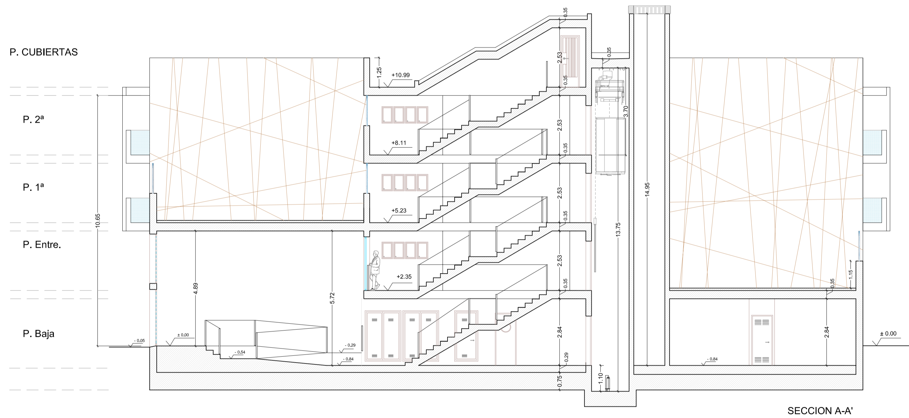
SECCION A-A'
